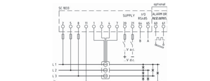
Q52D3H... per linea trifase 3 o 4 fili / for three-phase 3 or 4 wires system su linea a 3 fili non collegare il morsetto 11 / for 3 wires circuit do not wire terminal no 11
