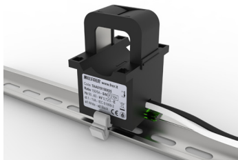
Fissaggio su guida DIN DIN-rail fixing
