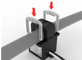
Fissaggio su primario Primary cable fixing
